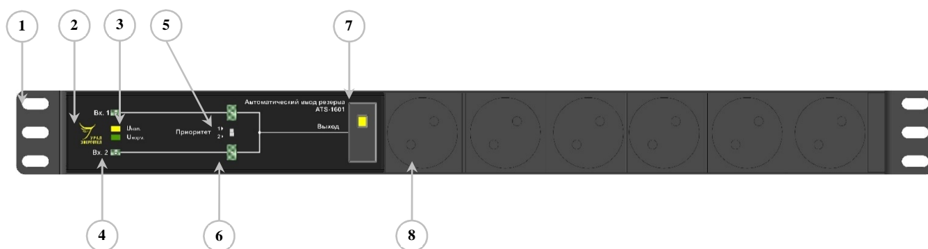
Рисунок 1 – Электронно-механический АВР ATS-1601(Р), передняя панель:
