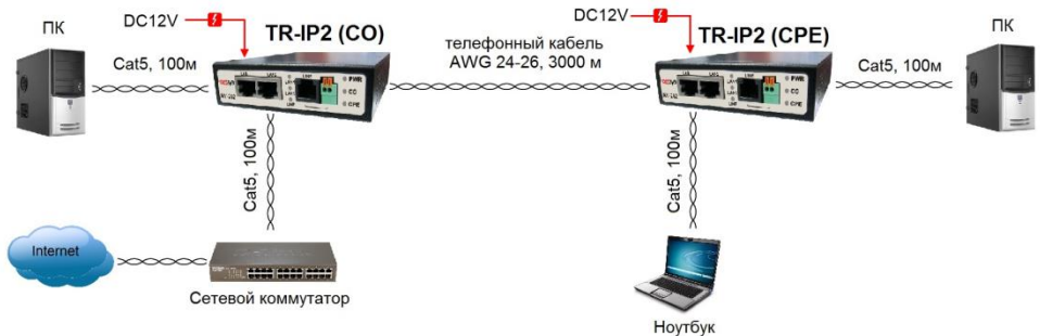
Рис. 6 Схема подключения TR-IP2 (CO) и TR-IP2 (CPE) для организации удаленных рабочих мест.
